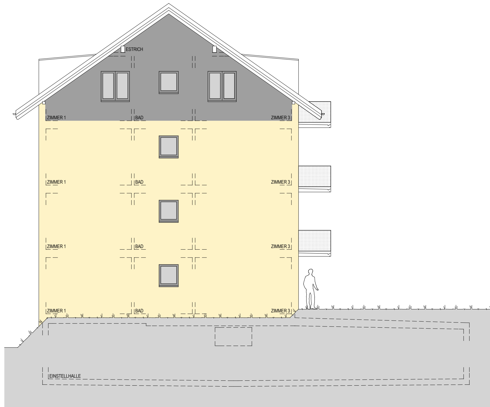
NORD FASSADE
