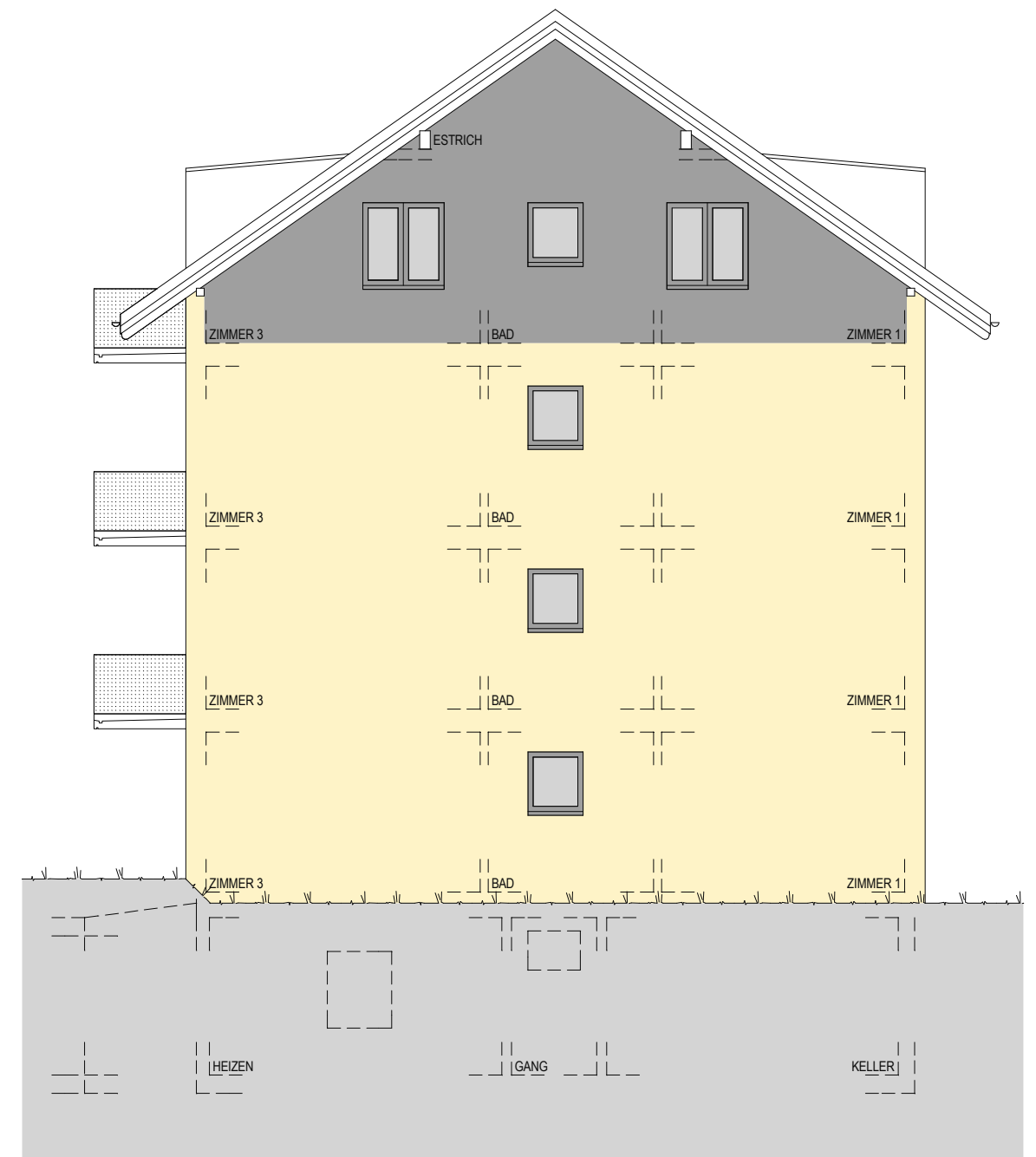
OST FASSADE
